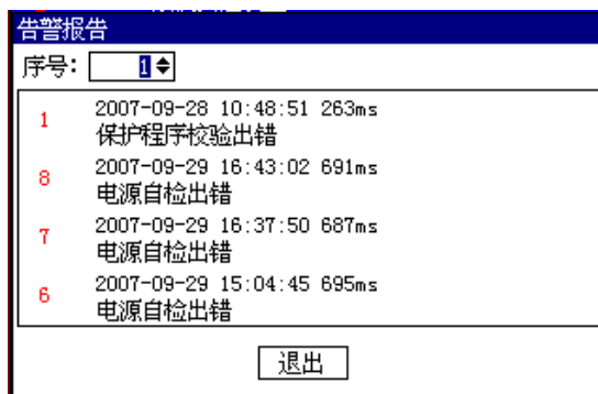
图 12-3-7-3 查看告警记录的窗口示例
