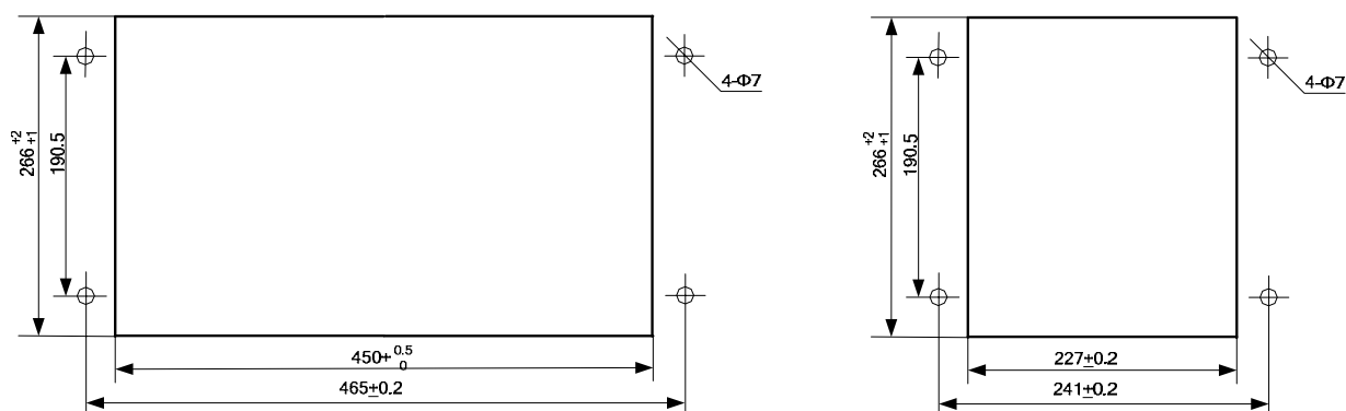
图 7-2 FCK-851 的开孔尺寸(左图为 FCK851/1-2 右图为 FCK851/3)
