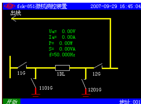
图 12-1 装置的主界面
