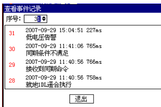
图 12-3-7-2 查看事件记录的窗口示例
