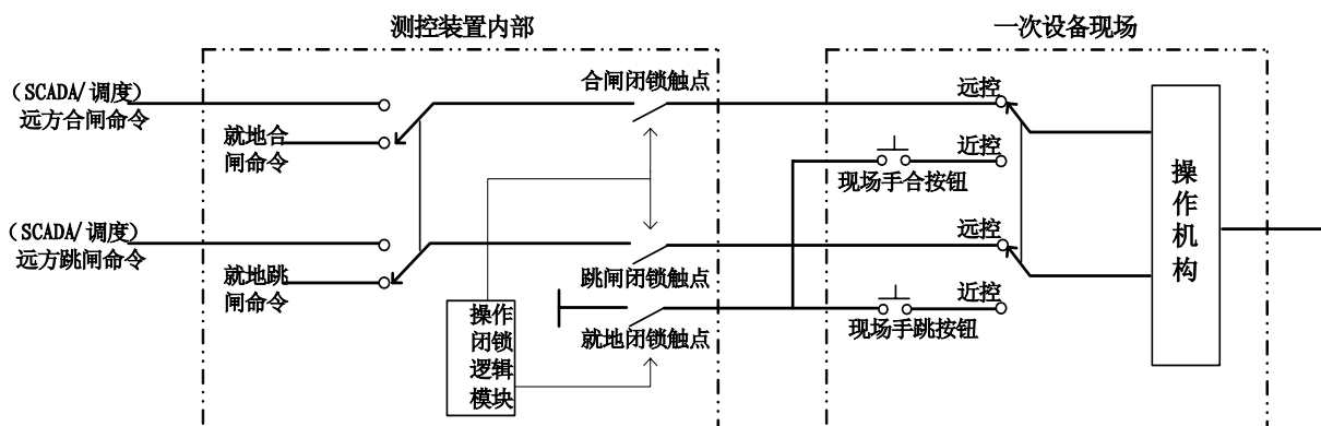
图 5-3 刀闸就地操作闭锁示意图
