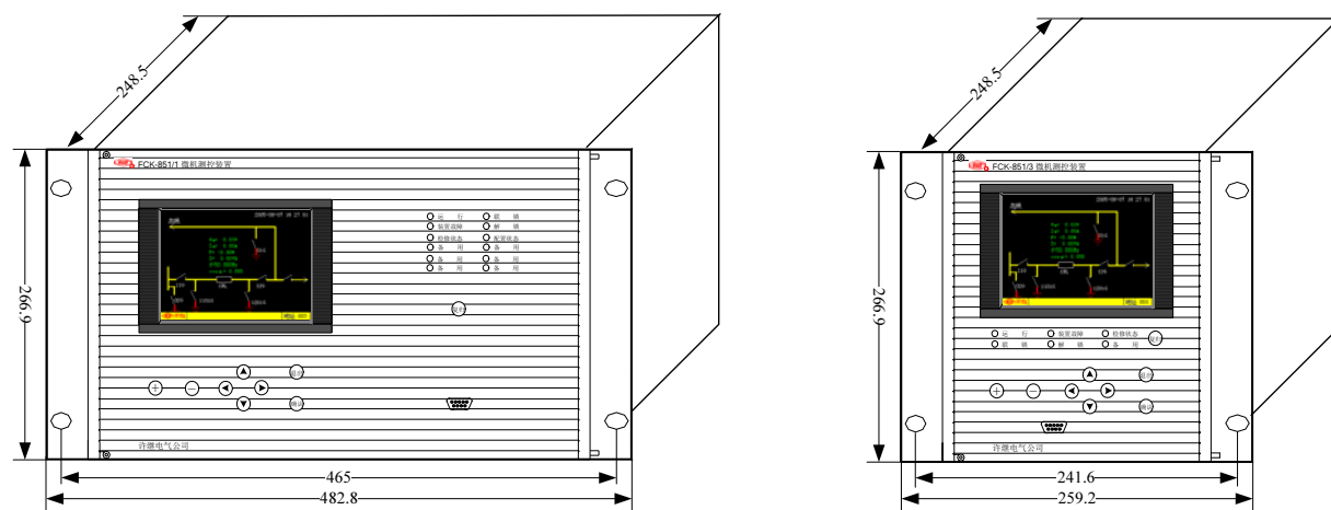
图 7-1 FCK-851 的外形尺寸(左图为 FCK851/1-2 右图为 FCK851/3)
