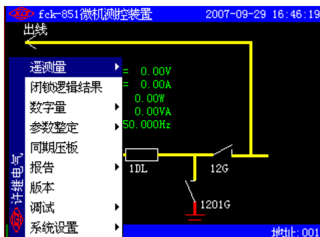
图 12-3 弹出固定菜单的主界面
