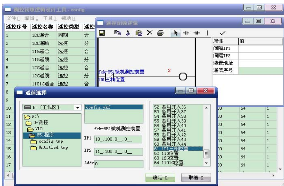
图 2 闭锁逻辑一键配置工作界面
